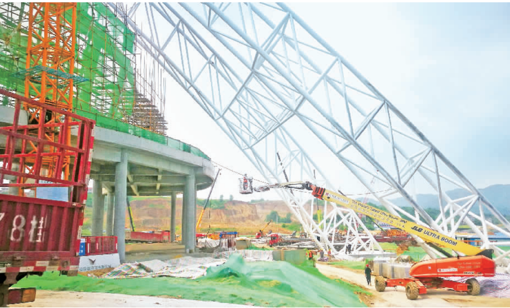
安康市体育馆(田径场)是承办第十四届全国运动会武术散打项目的比赛场馆。该项目位于汉滨区建民办长春路,作为安康市体育运动公园(江北体育运动中心)的子项目,占地160亩,建筑面积36441.34平方米,设计采用拱支网壳结构形式,地上局部4层,总座席5051座;足球田径场17031平方米,包含400米标准跑道、足球场及其他田径设施。项目概算总投资4.88亿元,截至今年4月底,项目累计完成投资3.65亿元,完成主体封顶。图为工人们正加紧体育馆钢结构施工。
